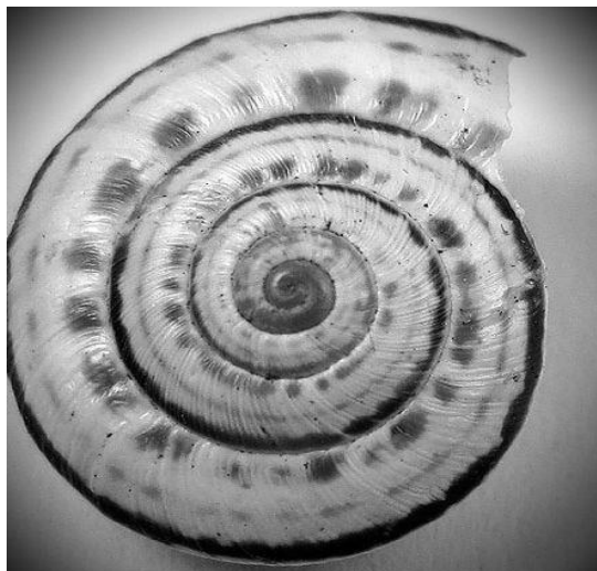
Fig. 13. Modèle pour l'étude de la spirale logarithmique, dite « de croissance ». Dans son évolution on observe une augmentation de sa taille. Elle grandit dans le sens horaire et se développe selon un mouvement centrifuge
