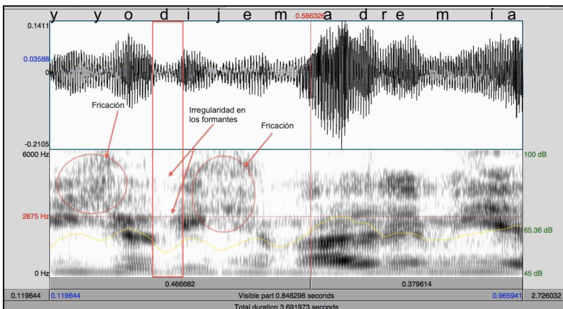
Fig. 2: Fragmento del sonido AN220401. Aproximante 2.
