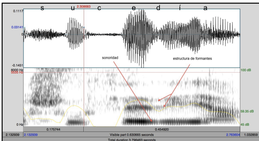
Fig. 1: Fragmento del sonido M175. Aproximante intervocálica (canónica).
