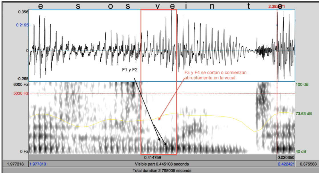
Fig. 3: Fragmento del sonido M417. Aproximante 3.
