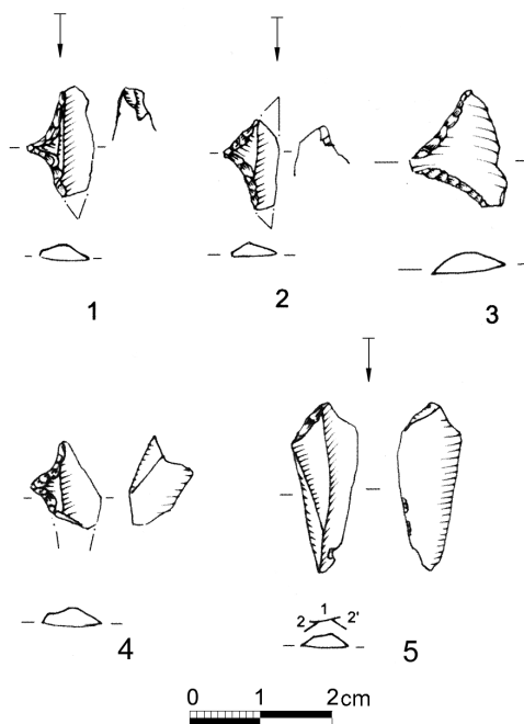
Fig.12. Mas de Sanç. Microlitos geométricos y microburiles
