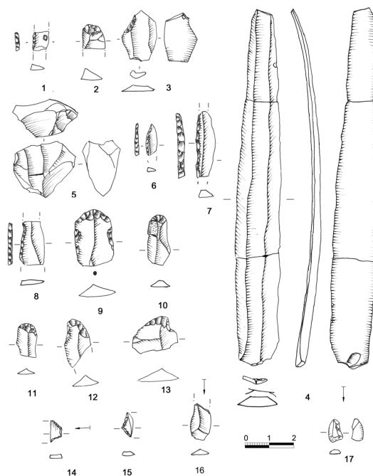
Fig.5. Cingle de l'Ermità. Industria lítica
