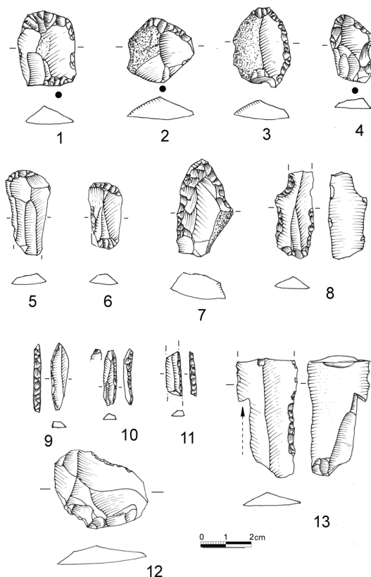
Fig.7. Cova del Trenc. Industria lítica
