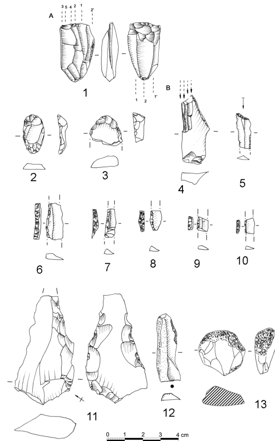
Fig. 3. Mas Blanc. Industria lítica
