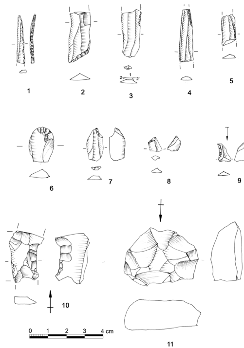
Fig. 9. Abric del Mas de Martí. Industria lítica del nivel 3
