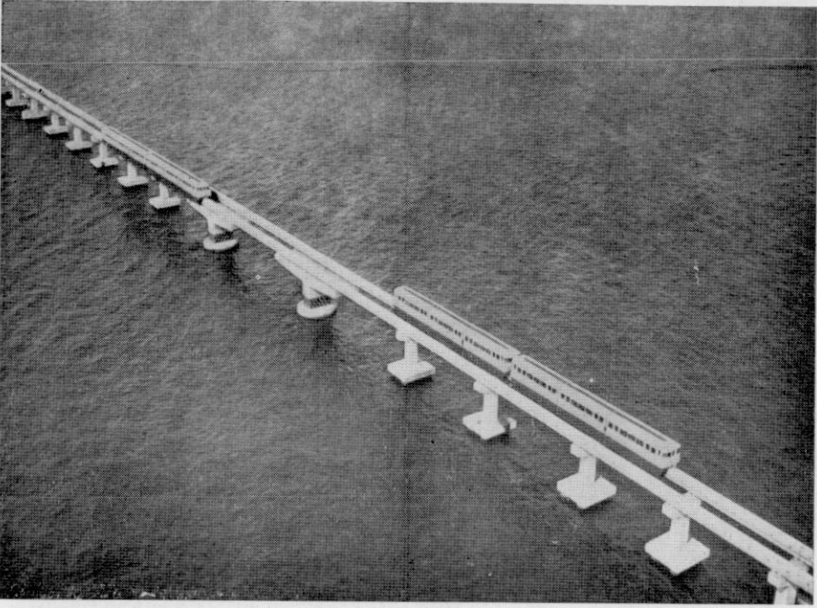
Fig. 1.—Monocarril elevado con neumáticos de Haneda (Tokyo), cruzando sobre la bahía.
