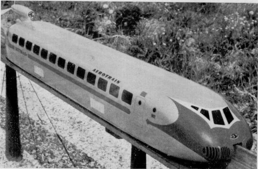
Fig. 2.—Maqueta del aerotrén Bertin, deslizante sobre colchón de aire y movido a turbopropulsión con hélice.
