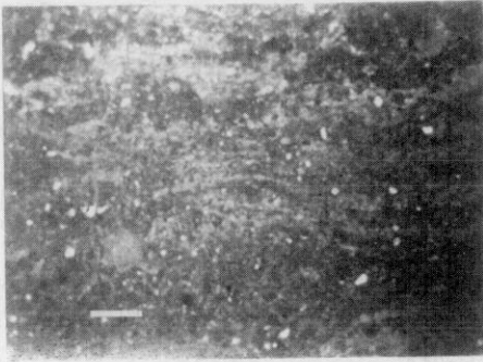
Fig. 2.- Microestructura laminar caracterizada por una alternancia de laminaciones claras y oscuras, generalmente onduladas, entre las que se depositan pequeñas partículas (terígenos). Escala 300 \mu\text{m} .
