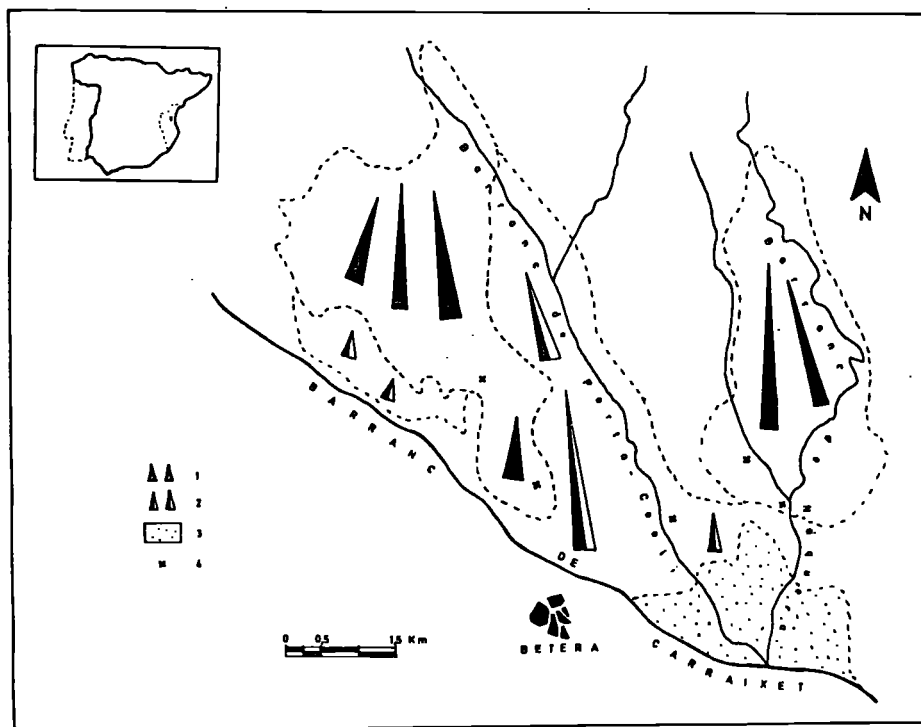
Fig. 1.- Esquema morfo-genético del sector del Barranc de Carraixet. 1) Nivel superior G_2-T_2 (Pleistoceno medio); 2) Nivel medio G_1-T_1 (Pleistoceno superior); 3) Mantos de arroyada holoceos; 4) Localización de los perfiles objeto de estudio.
