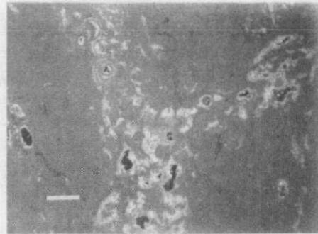
Fig. 7.- Pared de raíz micritizada. La materia orgánica no ha sido totalmente descompuesta quedando algunos filamentos en el interior de la misma; los huecos aparecen rellenos de microesparita. Escala 300 \mu\text{m} .
