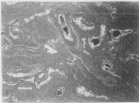
Fig. 6.- Huellas de raíces. Los huecos entre los restos vegetales aparecen rellenos de microesparita. En algunos de estos entramados de raíces es posible reconocer restos de tejidos de paredes vegetales que confirman su procedencia. Escala 300 \mu\text{m} .
